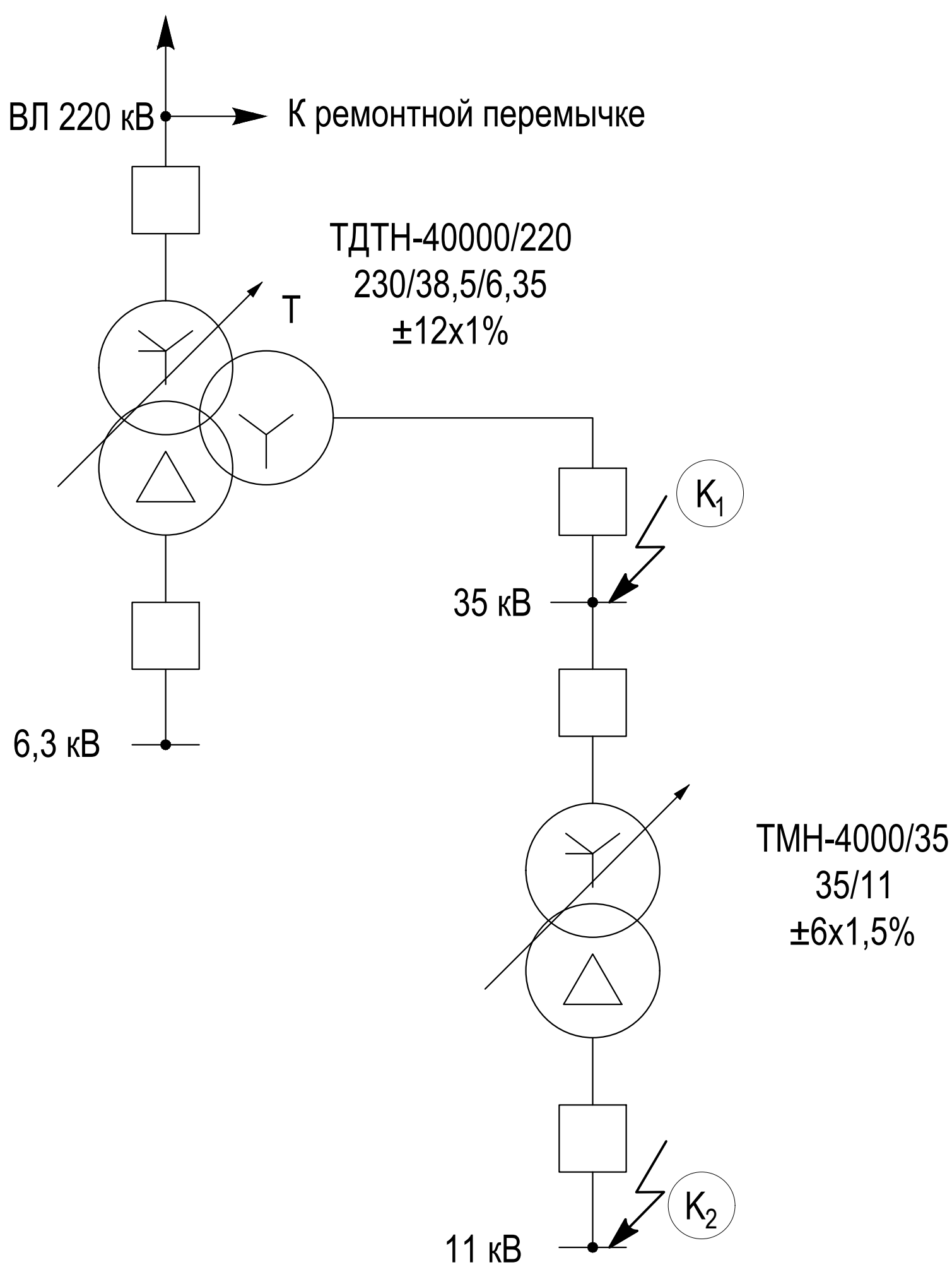
Поясняющая схема
