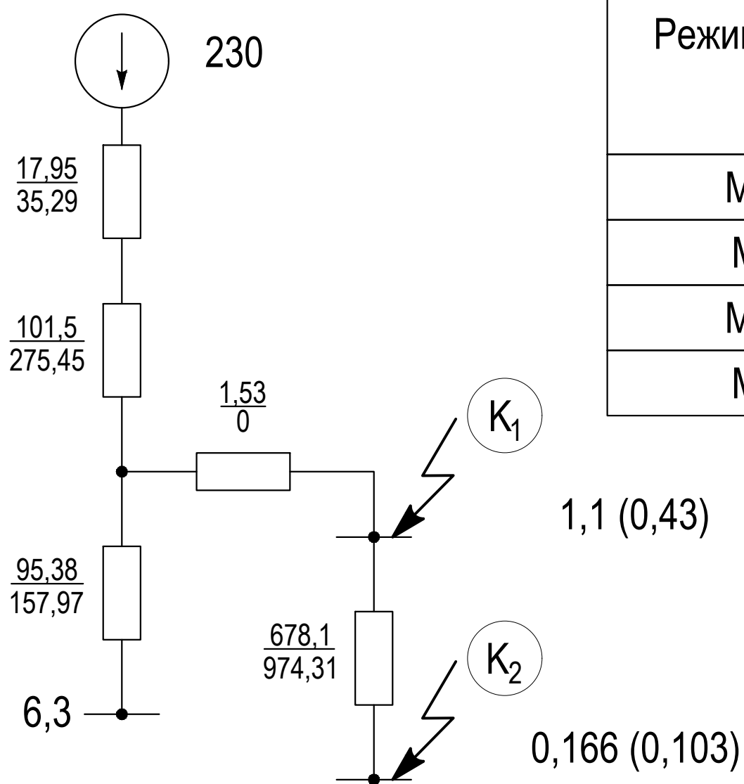
Схема замещения
